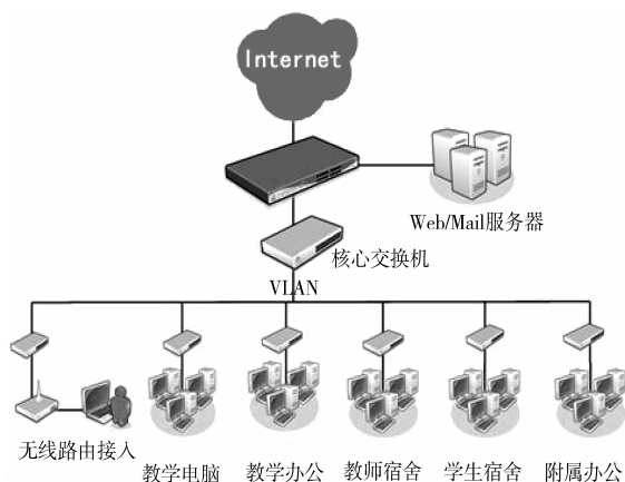
图1 校园网基本网络拓扑图
